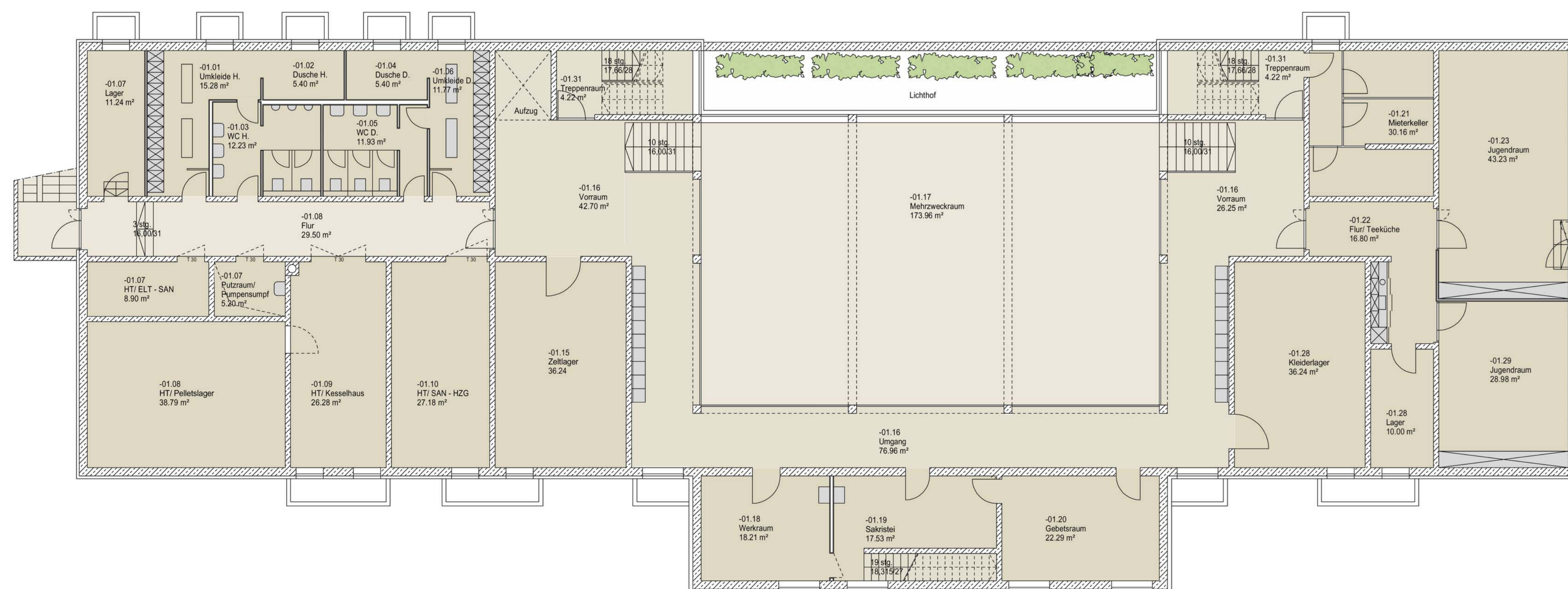
Untergeschoss
